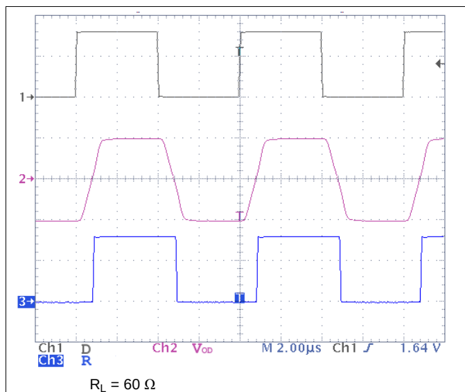
Figure 28. 65HVD72, 250 kbps
